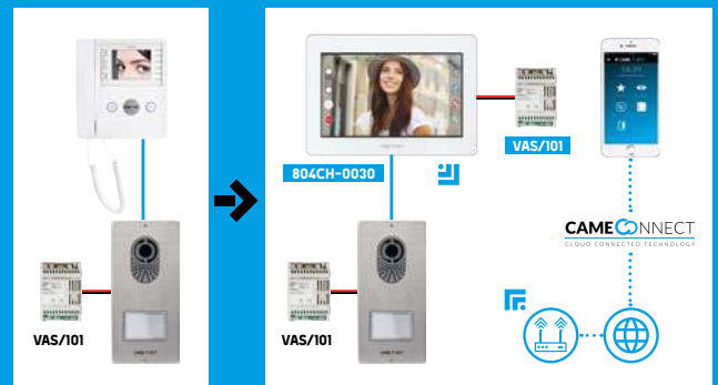
Alimentazione separata XTS e posto esterno
