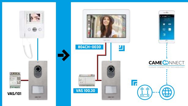
Alimentazione unica XTS e posto esterno
